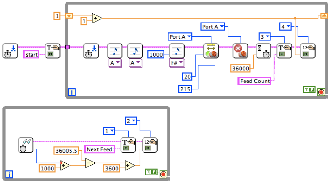
(LabView Code)
