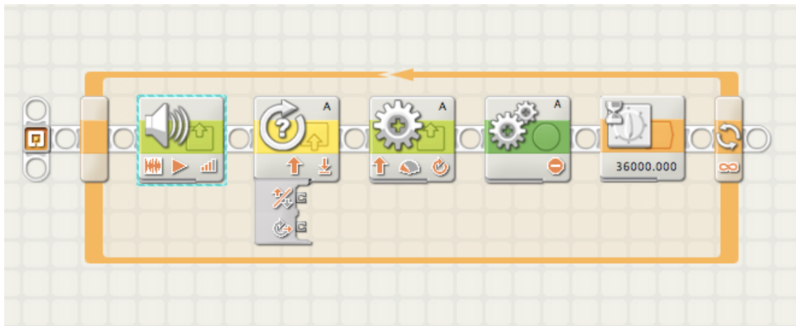
(NXT-G Code)
